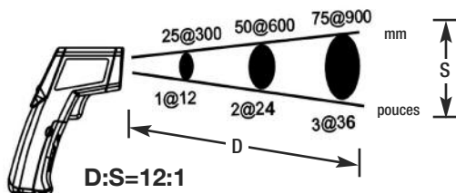
Fig. 3. Champ de vision du thermomètre IRT657
