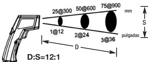
Figura 3. Campo de visión del termómetro IRT657
